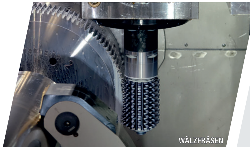
POWER SKIVING
